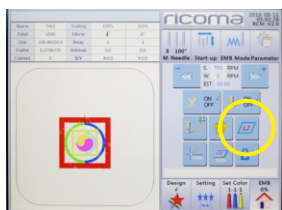
一键走框
